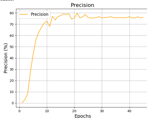
Gambar 3. Hasil precision
