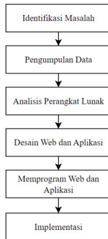
Gambar 1. Tahap penelitian
