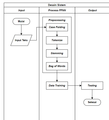
Gambar 2. Desain sistem
