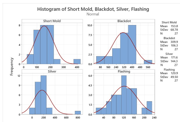
Gambar 3.3. Histogram Reject Periode Februari 2023
