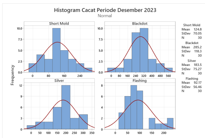
Gambar 3.1. Histogram Reject Periode Desember 2023
